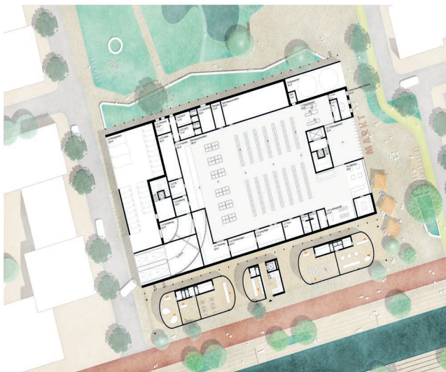
Grundriss Erdgeschoss
